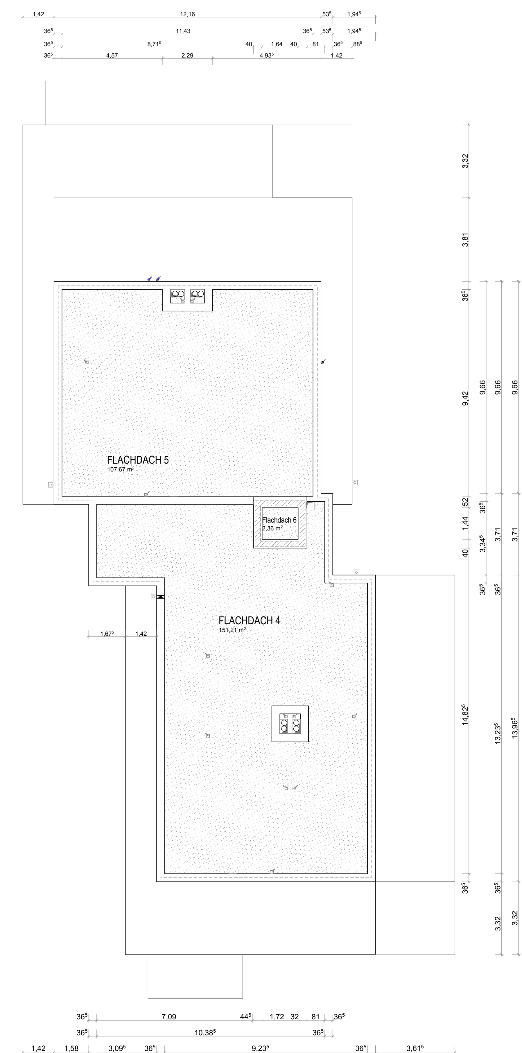
DACHAUSICHT
