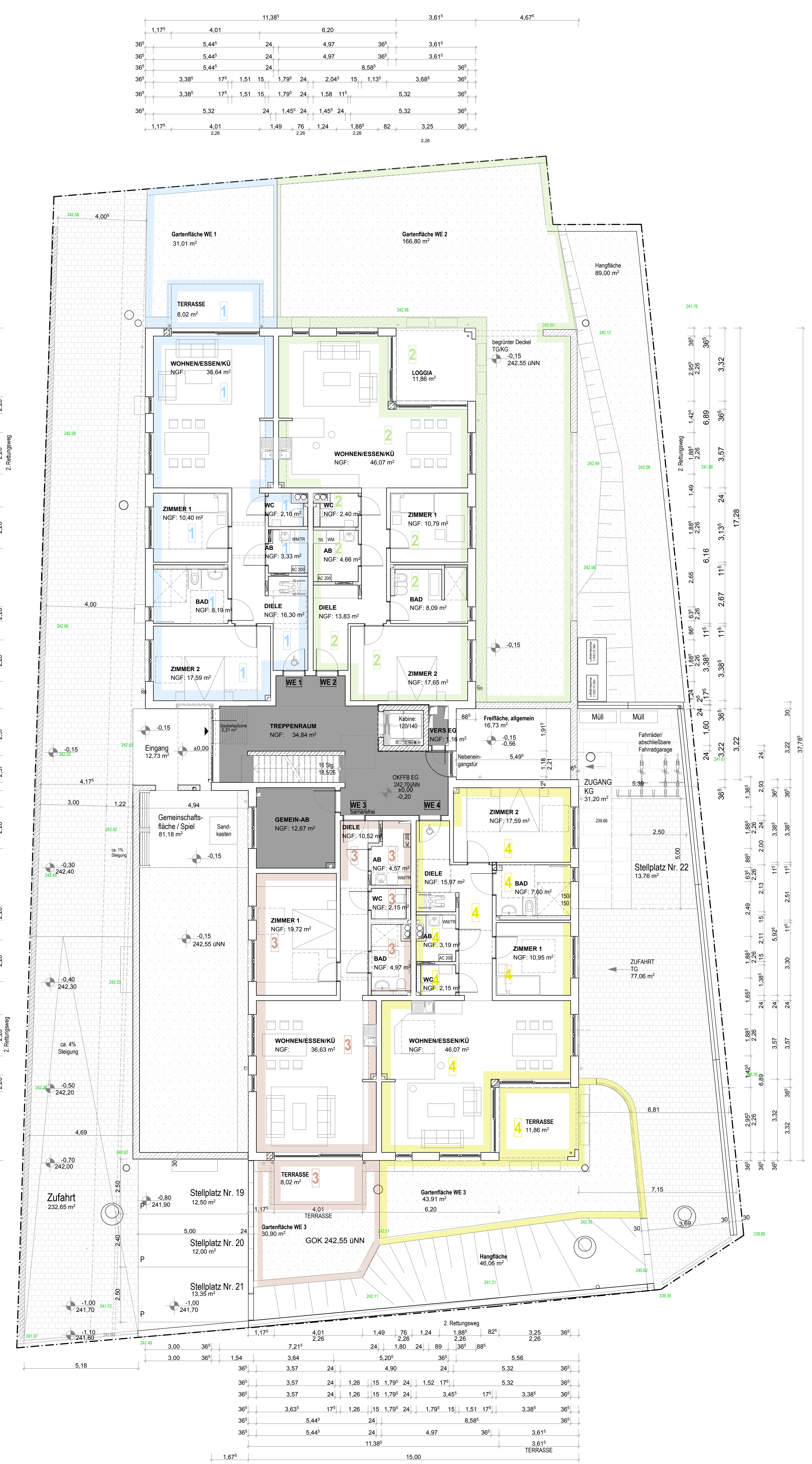
ERDGESCHOSS
